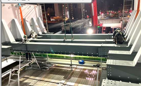
桁の組立作業を行っています
